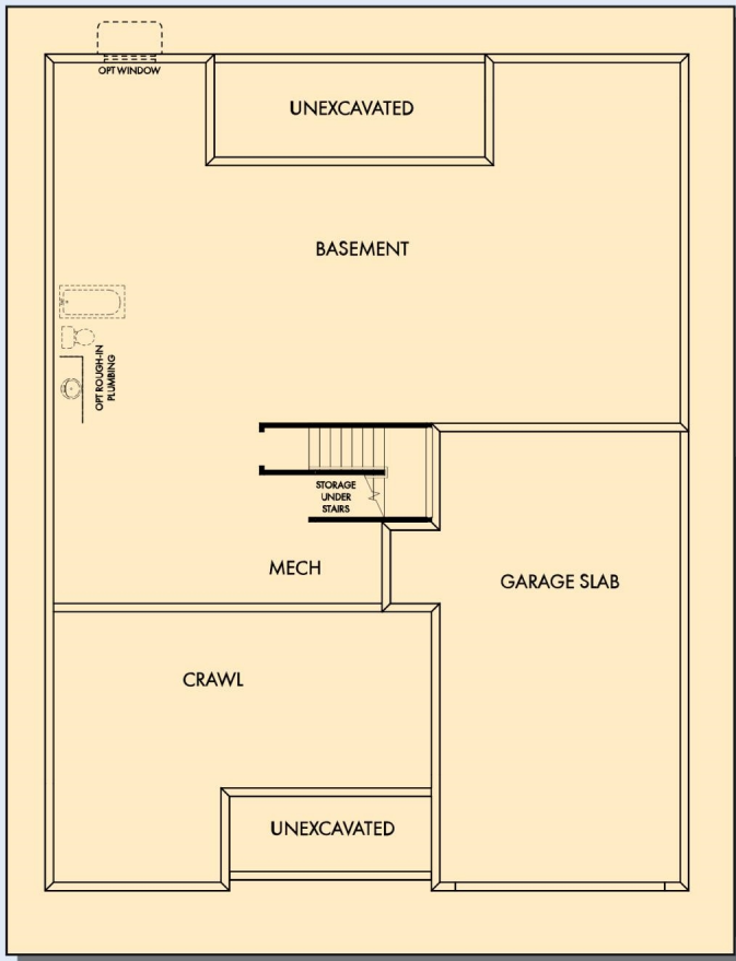
OPTIONAL BASEMENT
